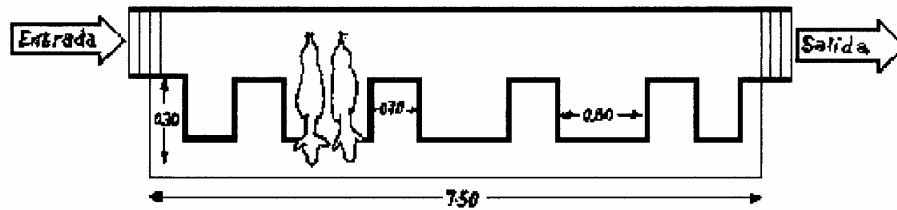
Sistema de Ordeño Tipo Tronera
