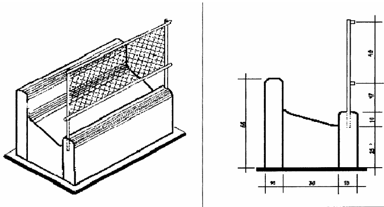
FIGURA 2. Vista general de un comedero y sus dimensiones
